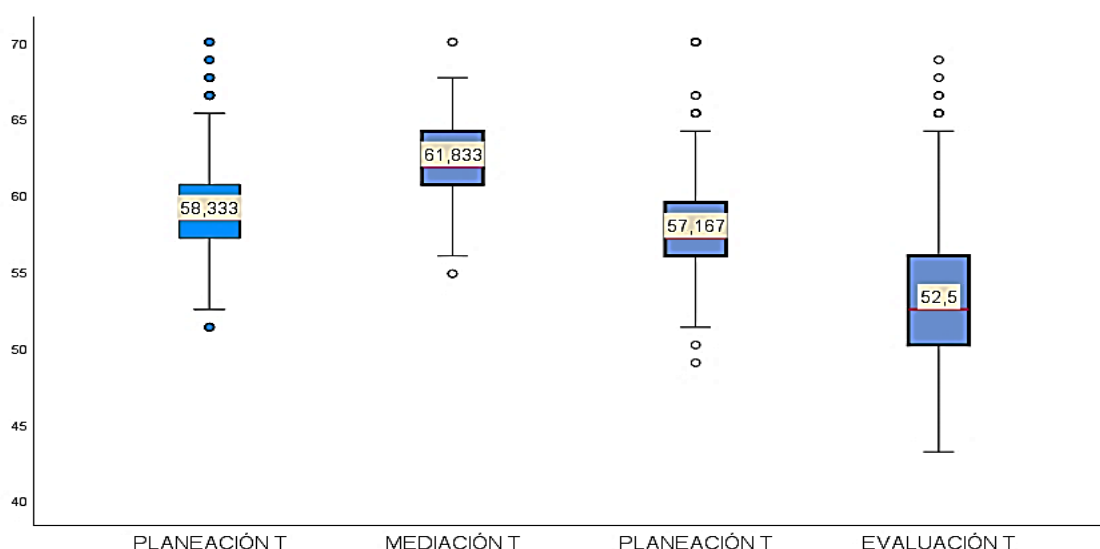
Gráfico 1. Generación de datos de planeación, mediación y evaluación. SPSS
