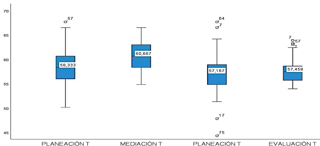
Gráfico 2: Generación de los datos de planeación, mediación y evaluación. SPSS.
